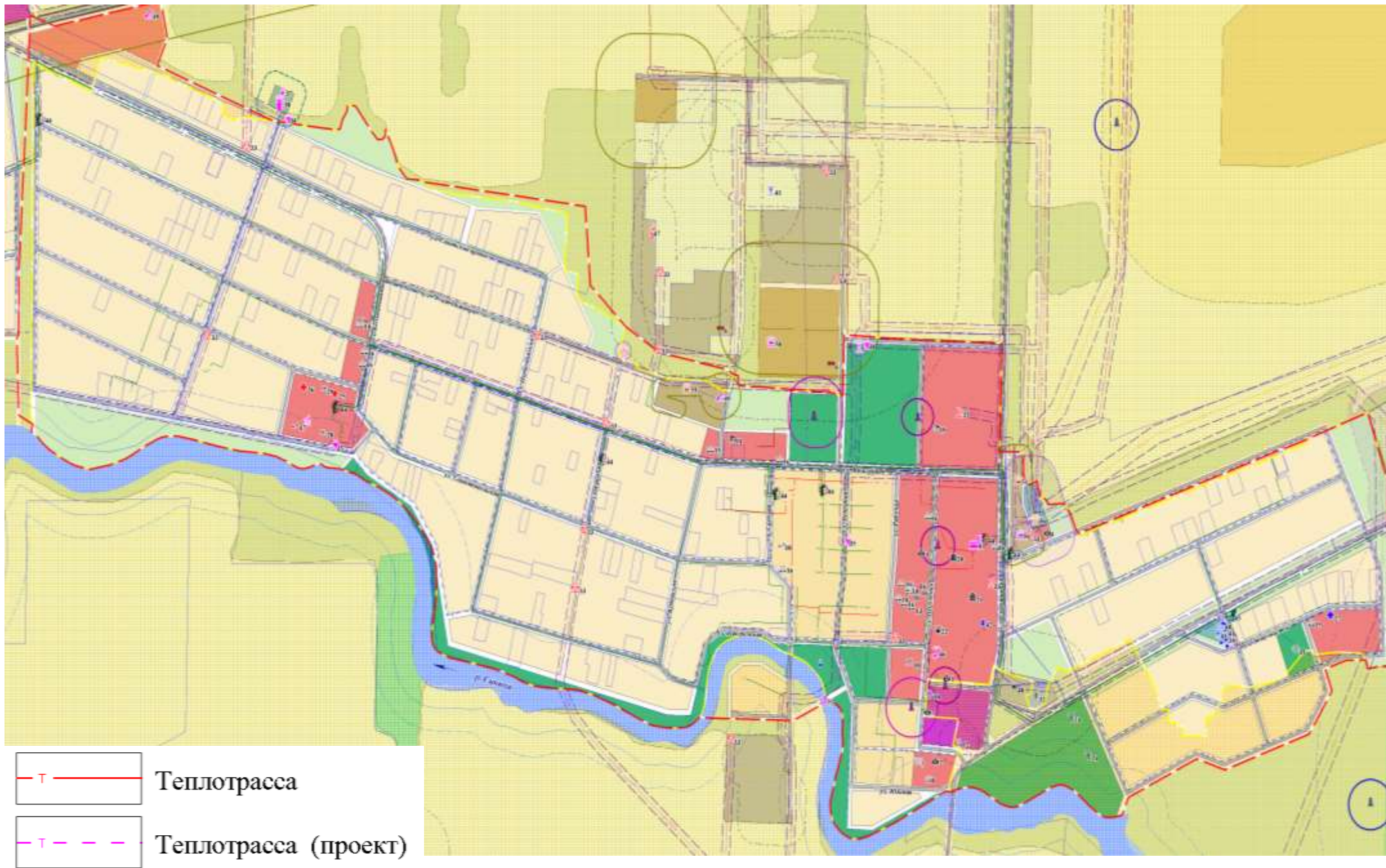
Поселок Кубань. Генеральный план перспективной схемы теплоснабжения
